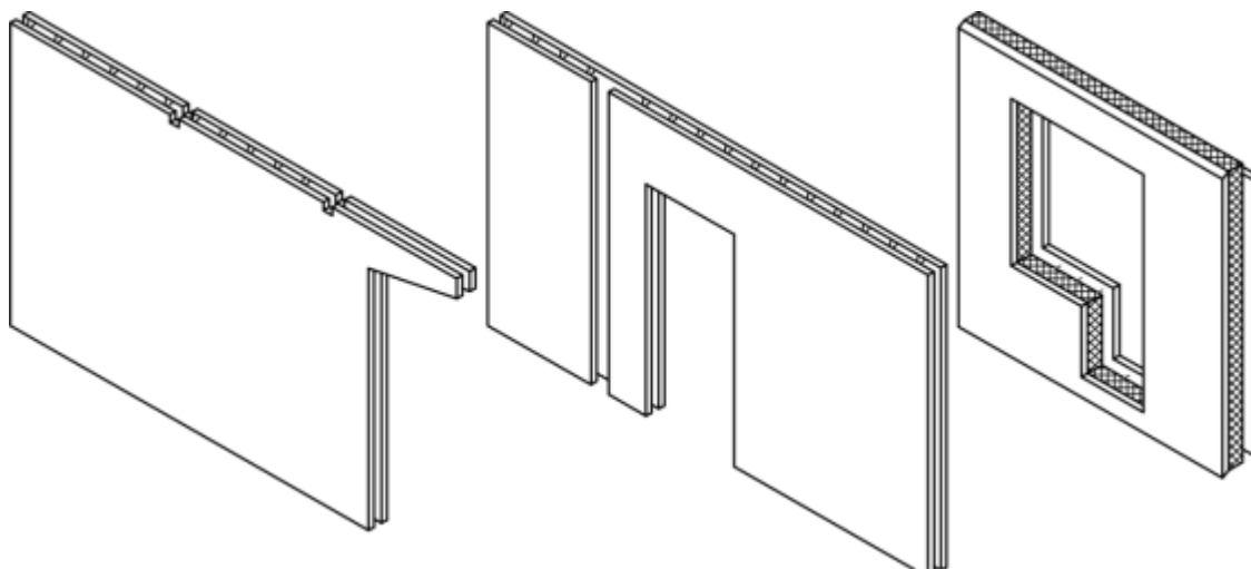
Рисунок 1 – Конструкция сборных железобетонных элементов несъемной опалубки перекрытия а), внутренних и наружных стен б)
