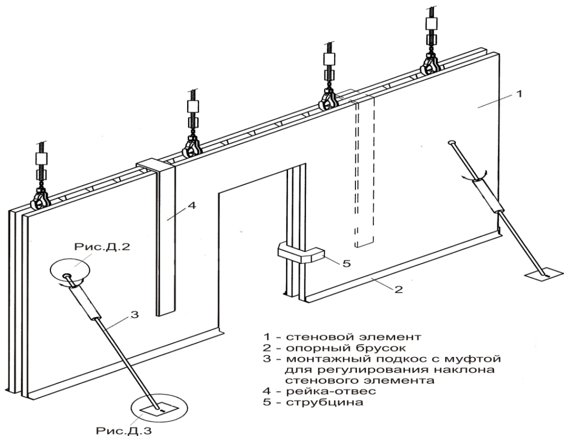
Рисунок Д.5 – Выверка стенового элемента при монтаже
