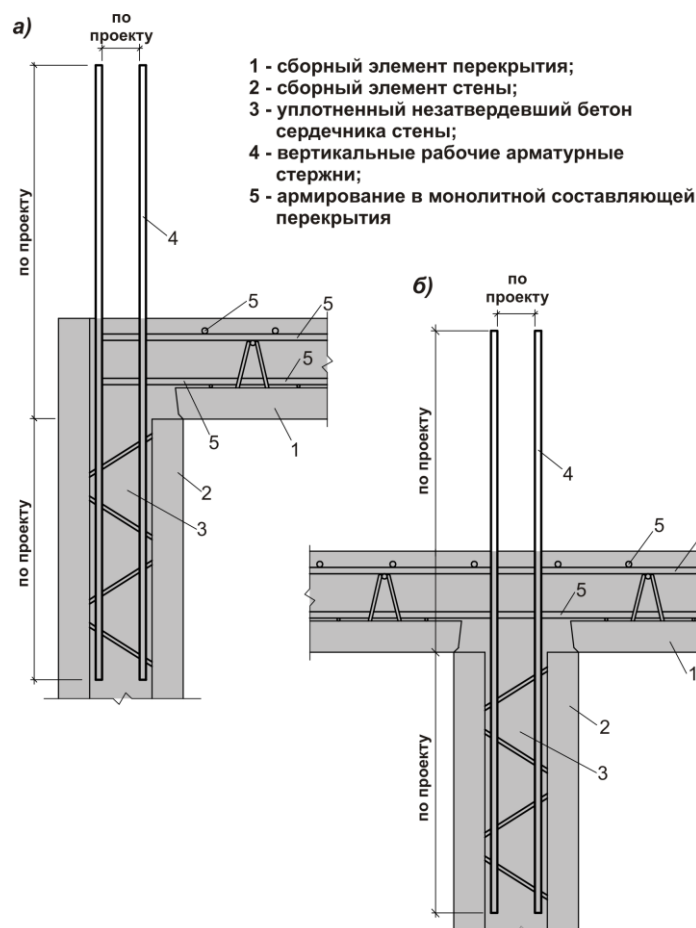
Рисунок 9 – Размещение вертикальных рабочих арматурных стержней в узлах сопряжения сборно-монолитных стен и перекрытий
